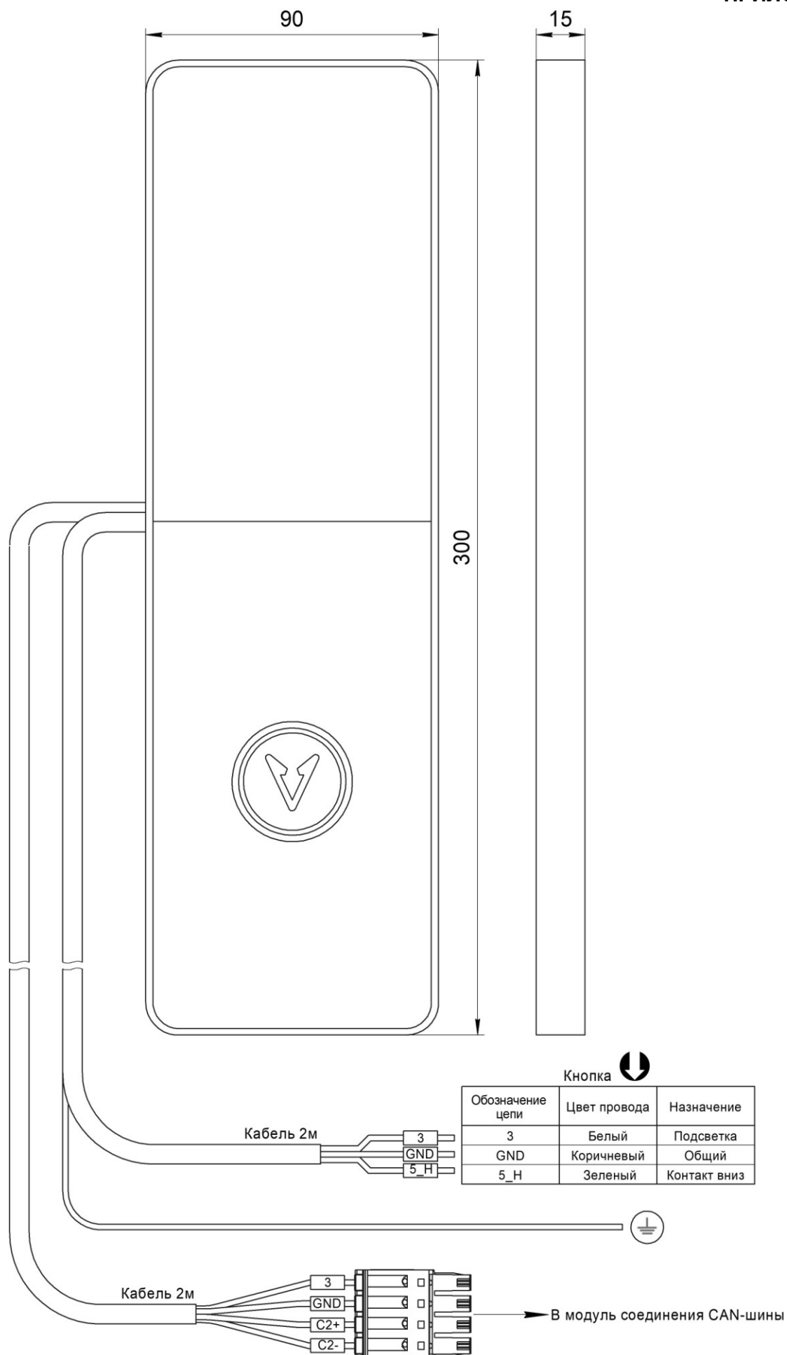
Рис.1 Внешний вид Вызывной пост ОПАЛ НШЕК.468381.056-01
